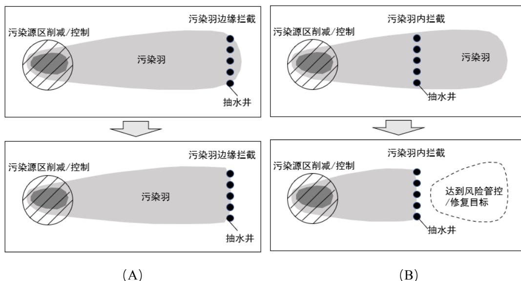
图3 污染羽控制策略抽水井布设示意图
